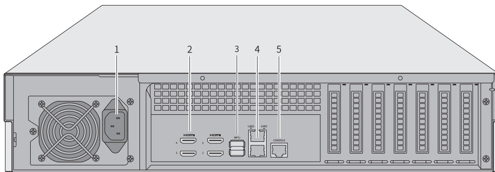
图1-3 TL-TUMS2600-N后面板示意图
